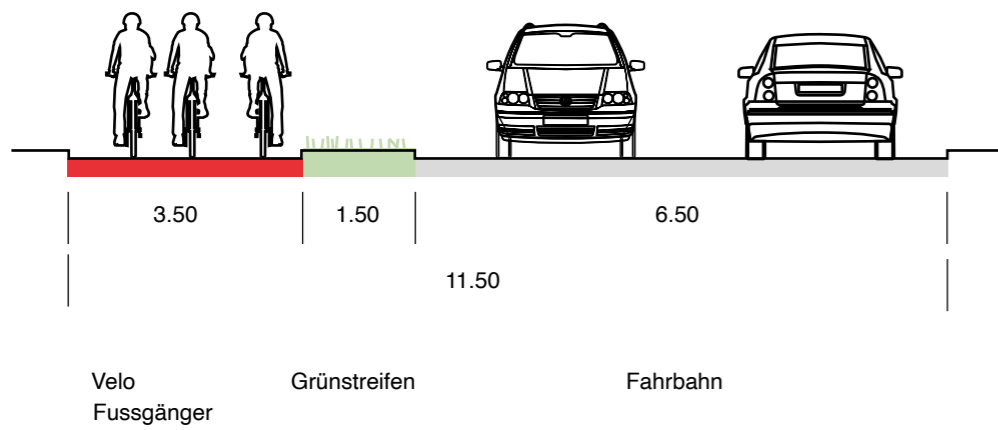
Querschnitt zukünftig
