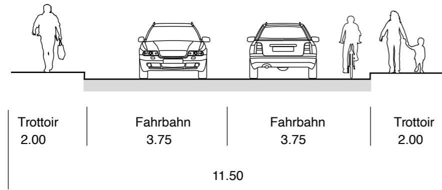
Querschnitt heute
