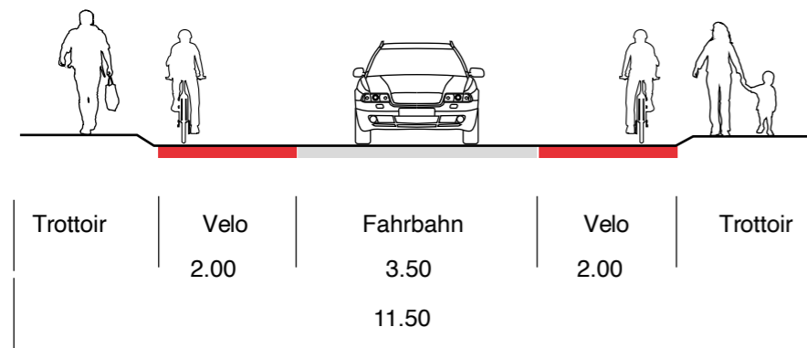
Querschnitt (überhöht)
